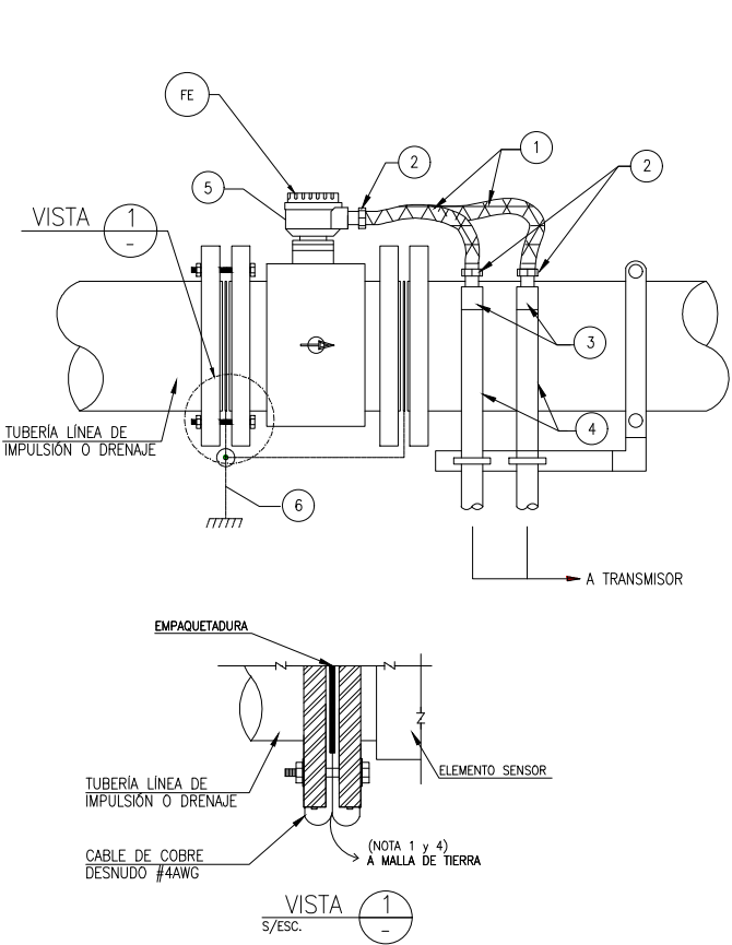
SENSOR DE FLUJO
