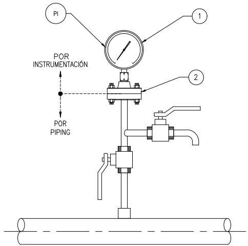
MANÓMETRO
