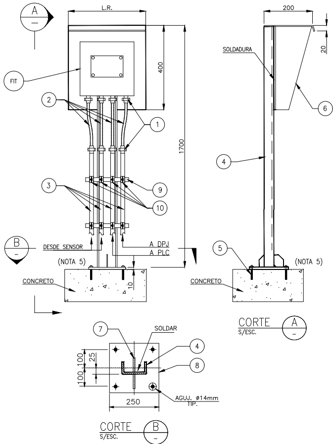
TRANSMISOR DE FLUJO
