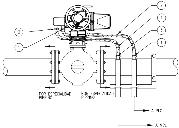
VÁLVULA MOTORIZADA
